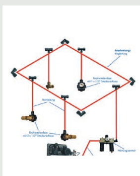
Rohrleitungen / Verbinder / Winkel / Verteiler
