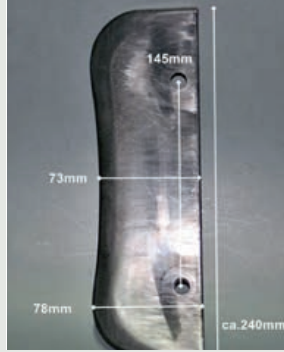
Kunststoffschutz für Abdrückschaufel
