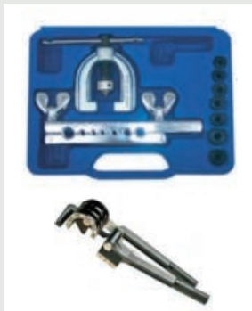
Bördelgerät – Rohrbiegegerät
