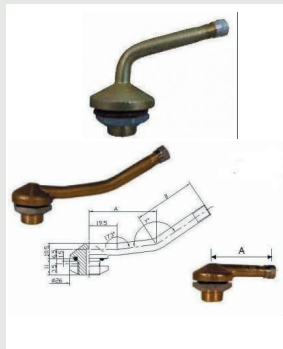
Ventilverlängerungen, LKW / Bus
